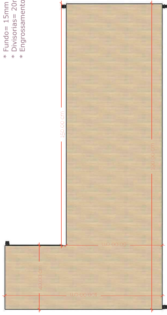
Vista Superior
