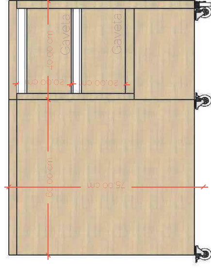
Vista Lateral
