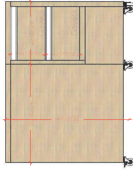
Vista Lateral
